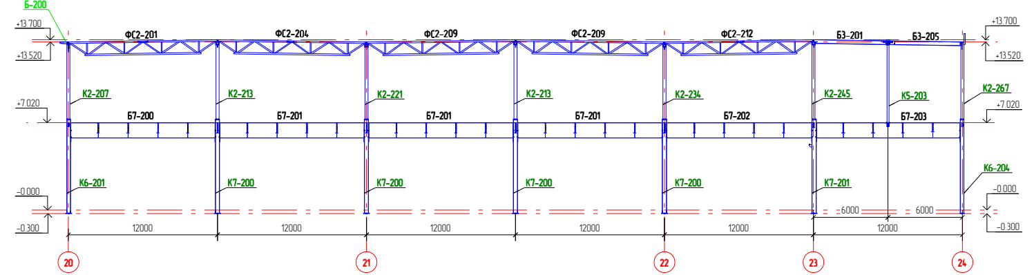
Разрез по оси Б
