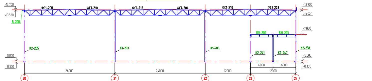
Разрез по оси Г
