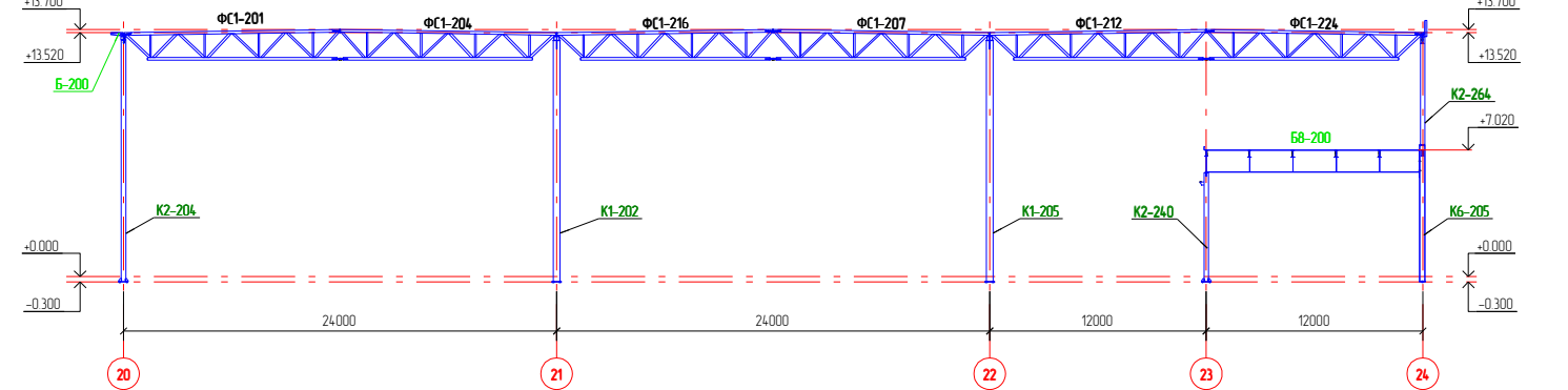
Разрез по оси Д
