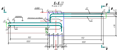
Вариант №2 анкеровки плиты с ростверком
