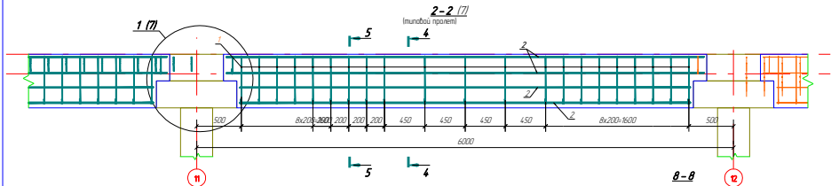
Вариант №1 анкеровки плиты с ростверком
