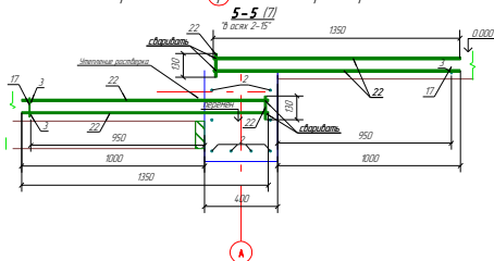
Вариант №2 анкеровки плиты с ростверком
