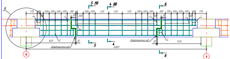
Узел 1 (8, 9) (схема анкеровки, армирование балки условно не показано)
