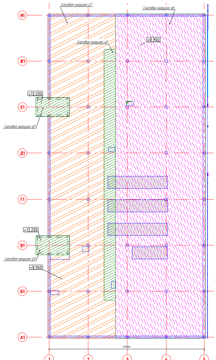
Снеговая нагрузка (покрытие АБК)
