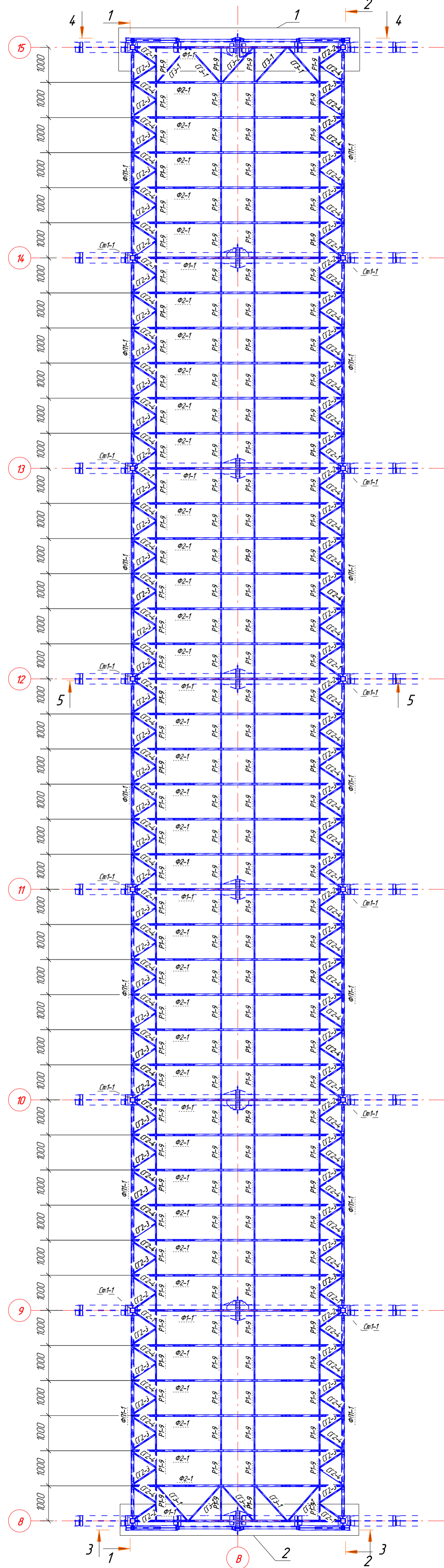
Схема расположения конструкций фонаря в осях В-15/В
